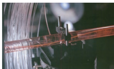
高速屈折率分布型ポリマー光ファイバー (High-speed graded index polymer optical fiber (GI POP))
