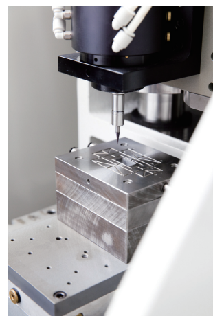
リニアモータ駆動小型超精密加工機
